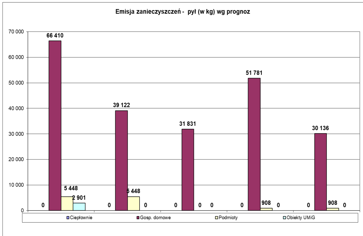
Wykres 7. Emisja zanieczyszczeń - pył (w kg) w latach 2019 - 2034
